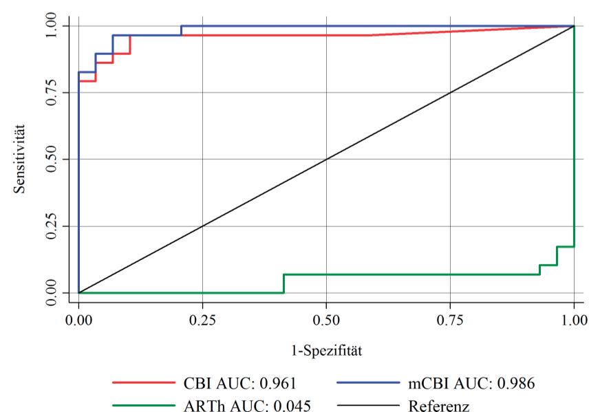
Abb. 2: Graphische Darstellung der Unterscheidungsgenauigkeit mittels der „Area under the curve“ (AUC) der untersuchten Indices. CBI: Corvis Biomechanical Index; ARTh: Ambrosio Relational Thickness = Dickenprofil der Hornhaut entlang des horizontalen Meridians (s. auch Abb. 1); mCBI: modifizierter CB = CBI ohne ARTh.
